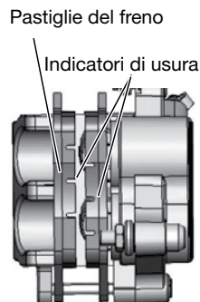
Freno anteriore
